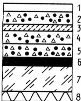
РИС. 2. Схема строения цветных фотоматериалов: 1 — защитный слой; 2 — синечувствительный слой; 3 — желтый фильтровый слой; 4 — зеленочувствительный слой; 5 — красночувствительный слой; 6 — противорефлексный слой; 7 — основа; 8 — противоскрепающий слой
