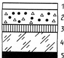
РИС. 1. Схема строения черно-белых фотоматериалов: 1 — защитный слой; 2 — светочувствительный слой; 3 — подслои (обычно у фотопленок) или баритовый (у фотобумаг); 4 — подложка, прозрачная бесцветная или подкрашенная противорефлексная (у фотопленок) и непрозрачная (у фотобумаг); 5 — противорефлексный слой
